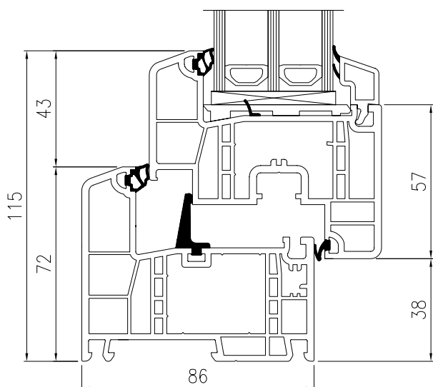
GENEO® Fenster
